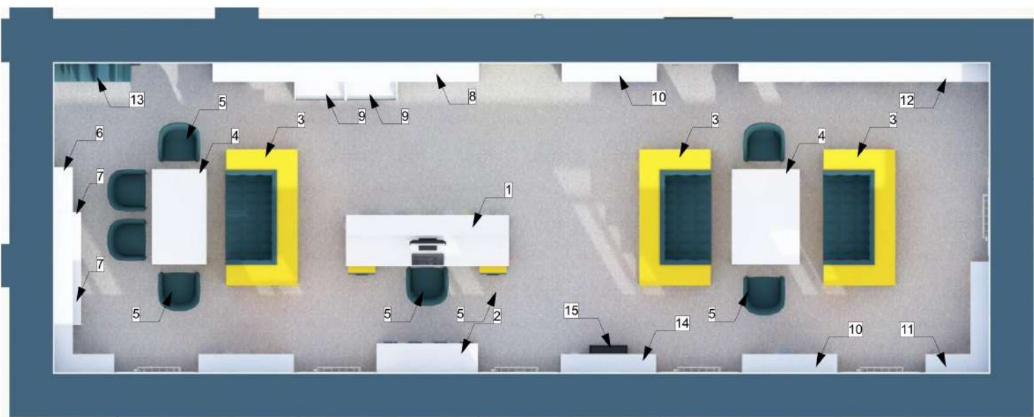
ПЛАН 1 ЭТАЖА. ЭКСПЛИКАЦИЯ ЭЛЕМЕНТОВ ОБОРУДОВАНИЯ.
